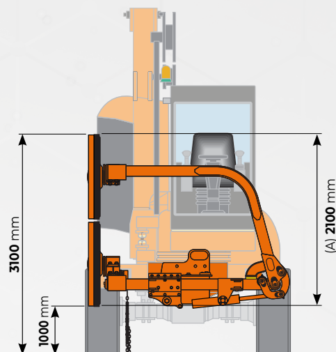
POSIZIONE DI TRASPORTO TRANSPORT POSITION
